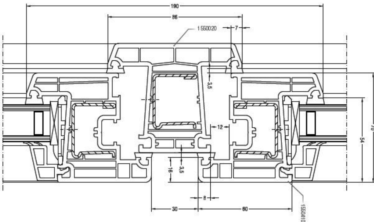
Sezione nodo Brillant 70 - 2 ante ( anta dritta )
